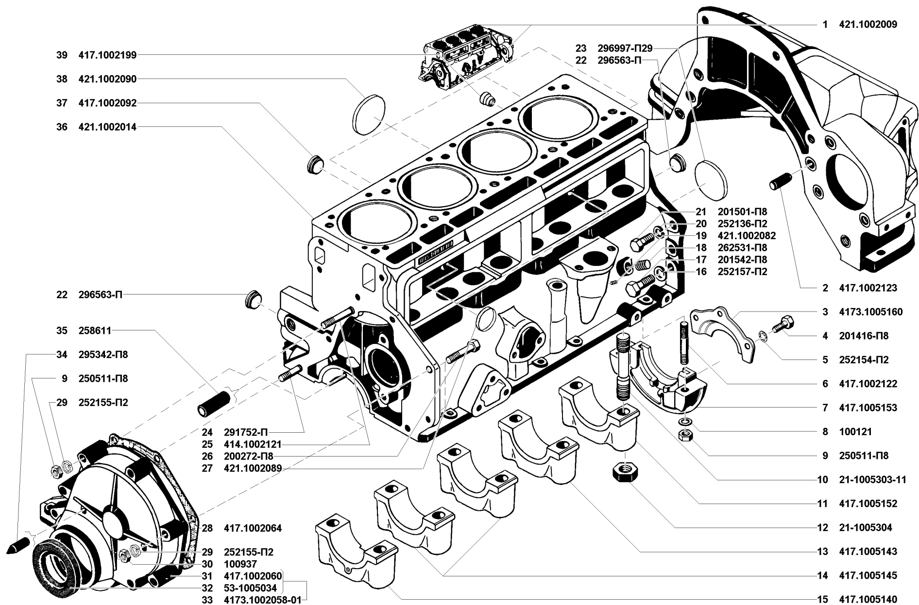
Рис. 5. Блок цилиндров двигателя (1002)/1
